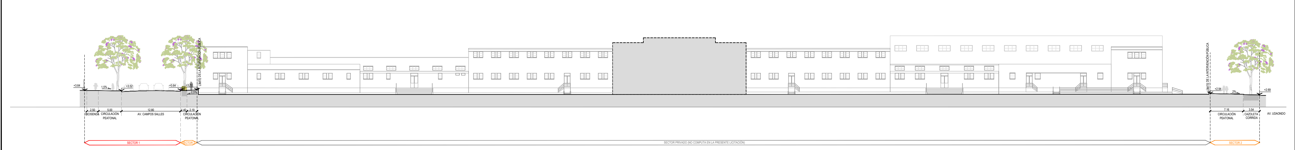
CORTE D-D Esc. 1:250
