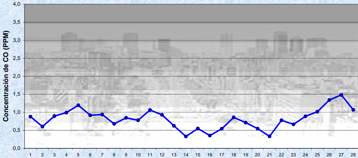
FEBRERO 2010 Concentración diaria de CO
