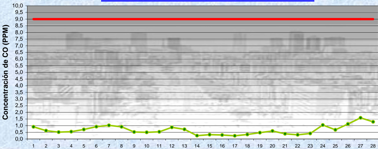
FEBRERO 2010 Concentración de CO- promedios de 8 hs
