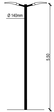
ESQUEMA DE COLUMNA Esc: 1:75
