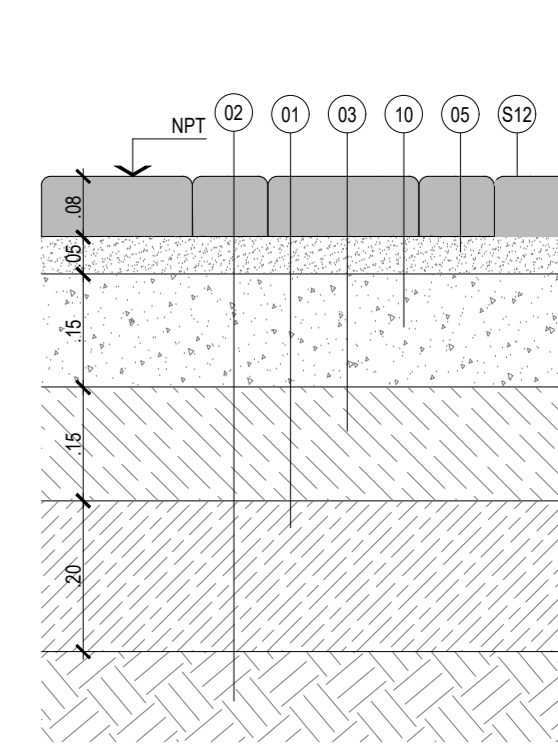
CORTE 1:10
