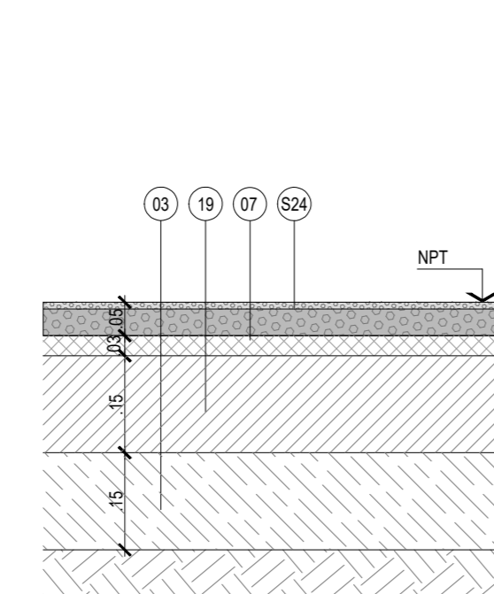
CORTE 1:10
