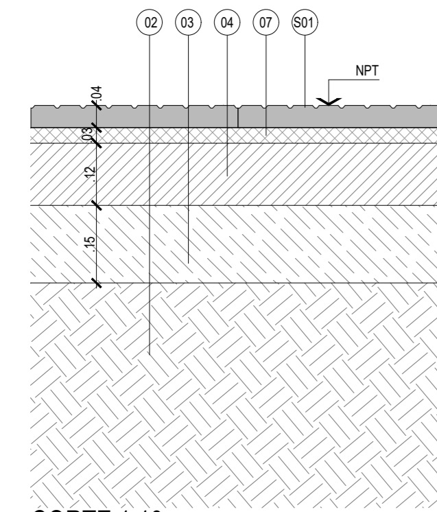
CORTE 1:10
