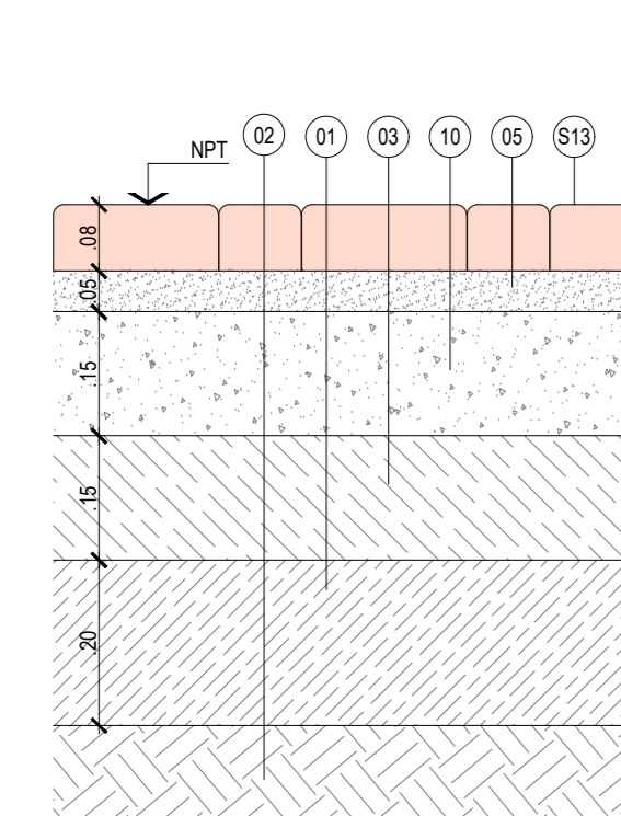
CORTE 1:10
