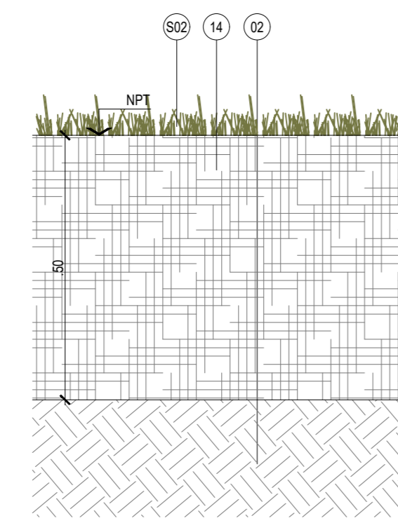
CORTE 1:10
