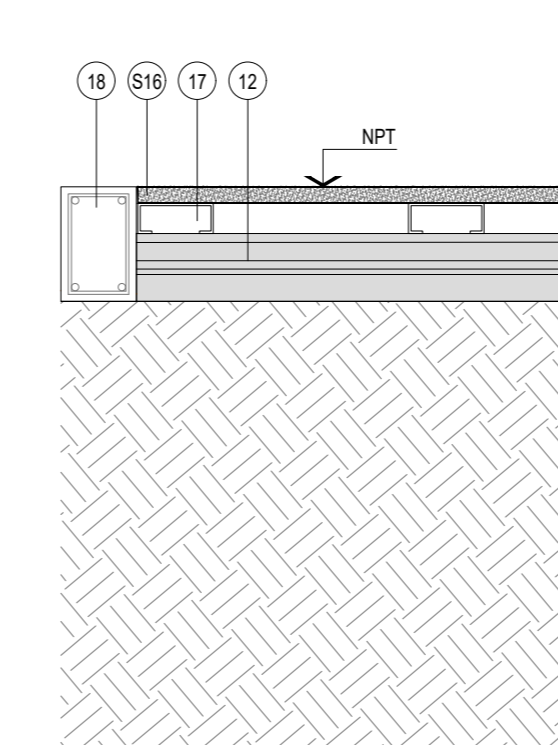
CORTE 1:10
