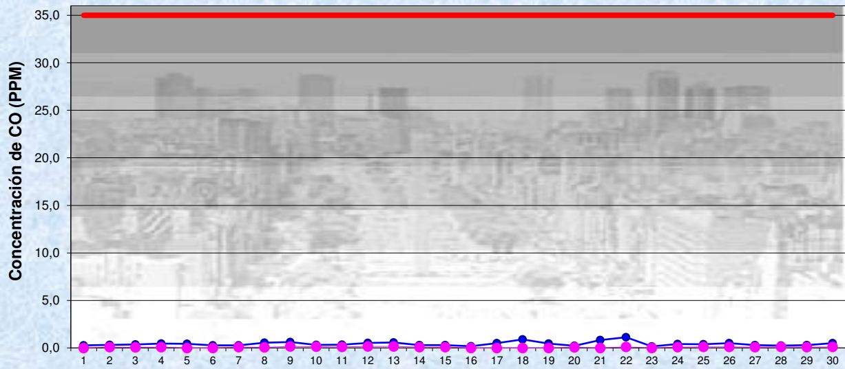
NOVIEMBRE 2018 Concentración de CO- Máximos y mínimos en intervalos de 1 hora
