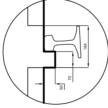
DETALLE A 1:10
