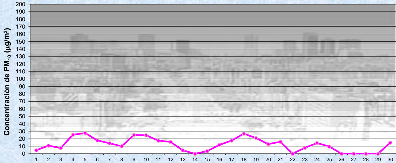
ABRIL 2024 Estación Pque. Centenario Concentración de PM 10 -Promedio de 8 Hs
