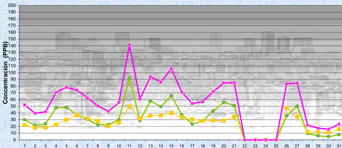
MARZO 2013 Concentración diaria ● NO ■ NO2 ◆ NOx Estación Parque Centenario
