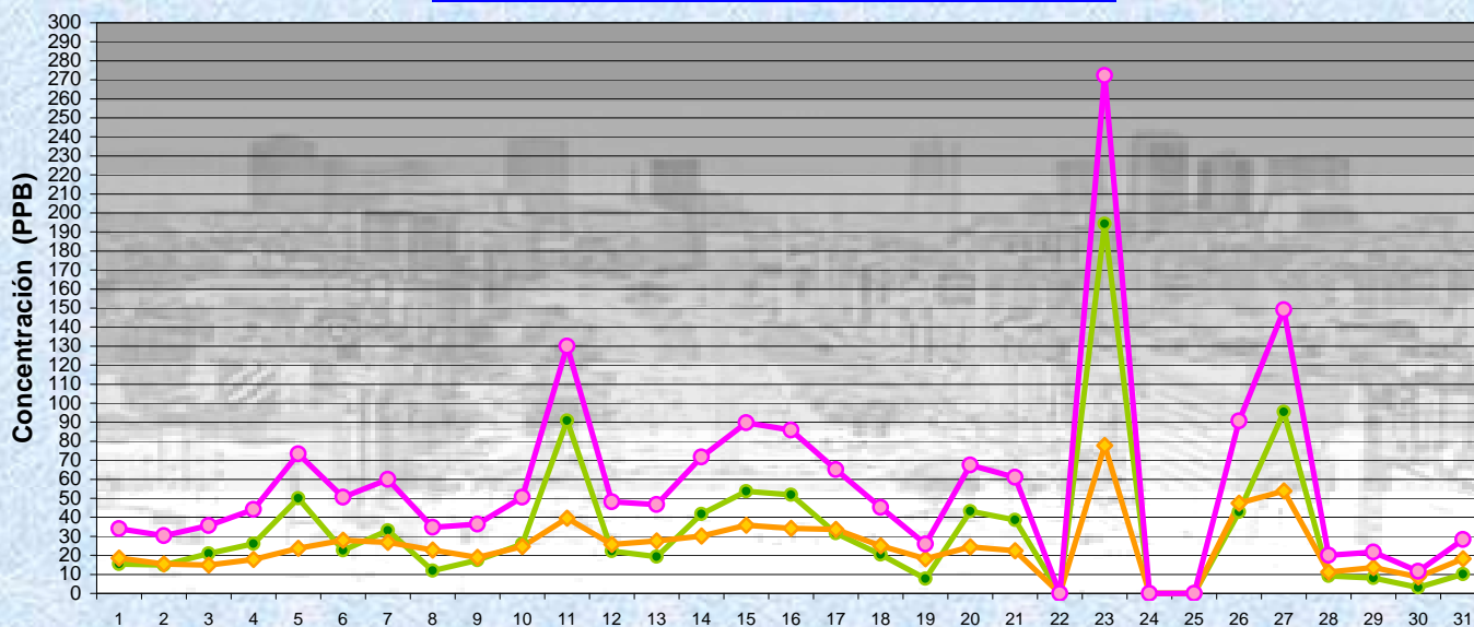
MARZO 2013 Concentración promedios de 8 hs De 0 a 8 Hs ● NO ◆ NO2 ◆ NOx Estación Parque Centenario
