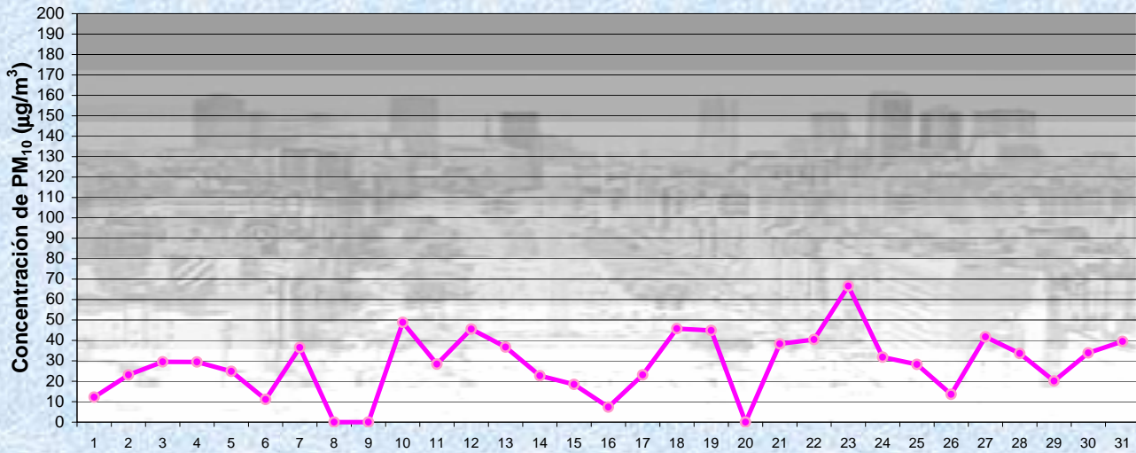
Estación Pque Centenario AGOSTO 2010 Concentración de PM 10 -Promedio de 8 Hs —●— PM10 de 8 a 16 hs
