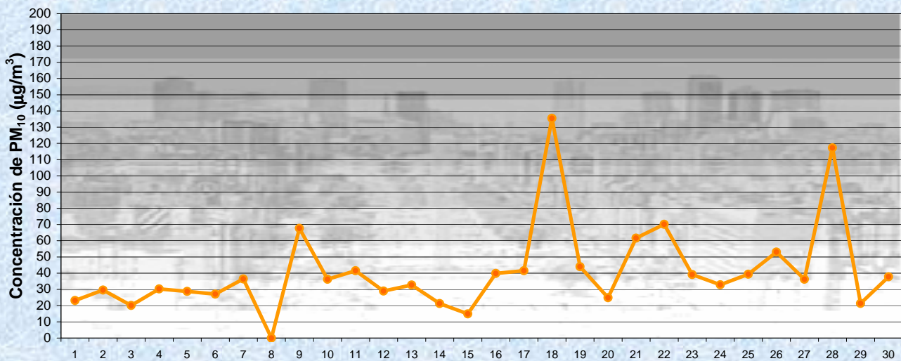
Estación Pque Centenario AGOSTO 2010 Concentración de PM 10 -Promedio de 8 Hs —●— PM10 de 16 a 24 hs
