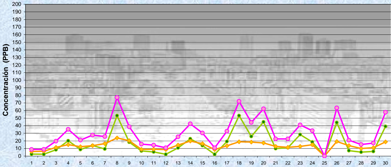
Estación La Boca ABRIL 2013 Concentración promedios de 8 hs De 0 a 8 Hs ● NO ◆ NO2 ◆ NOx
