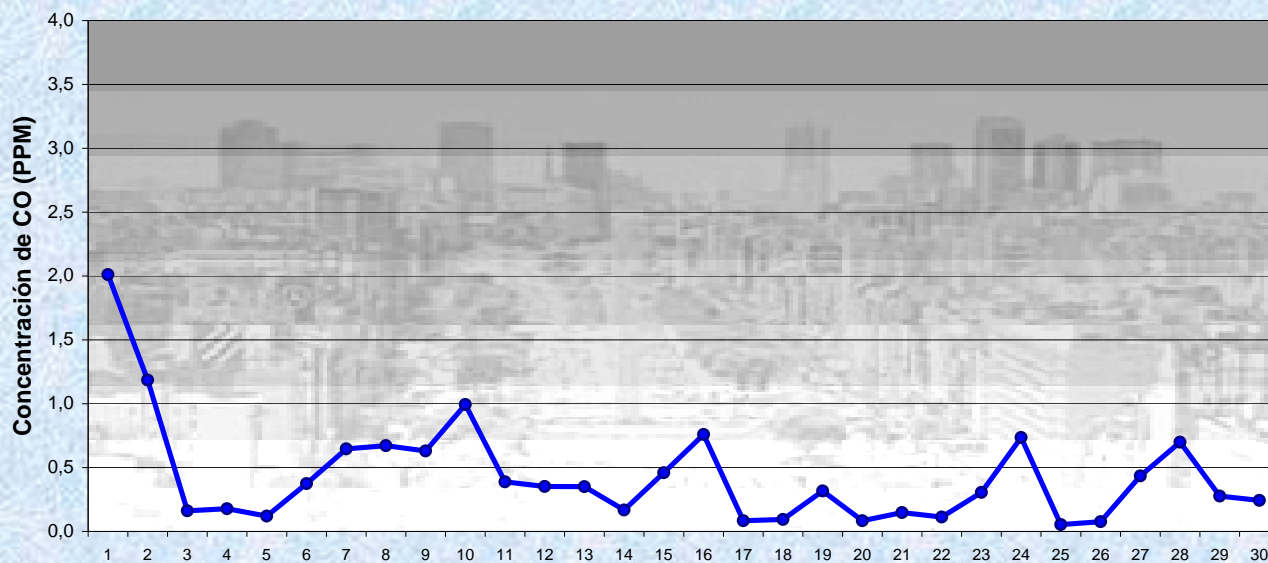
JUNIO 2011 Concentración diaria de CO
