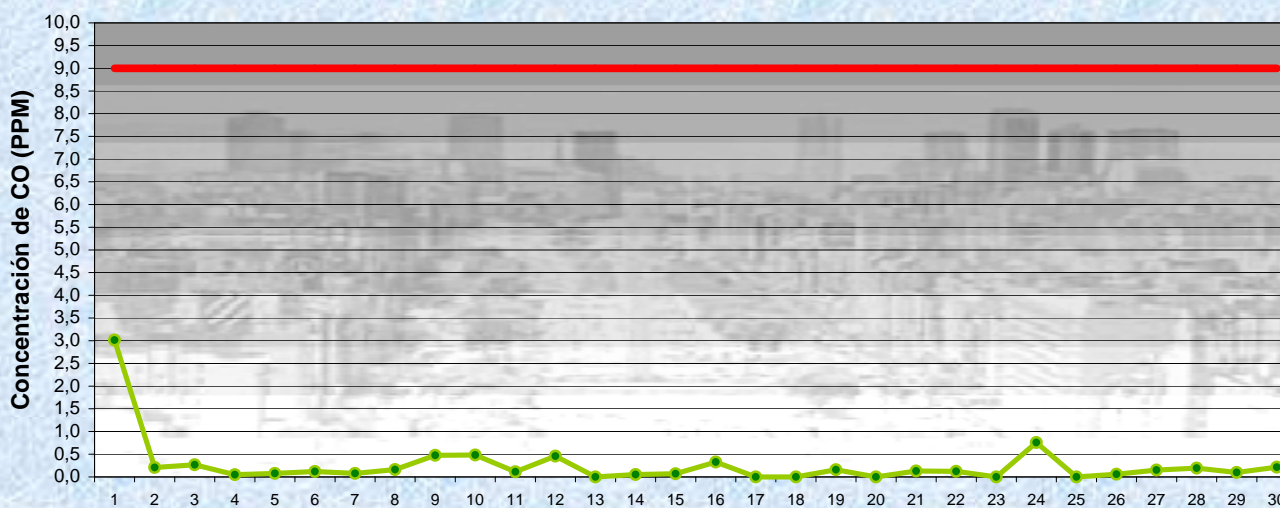
JUNIO 2011 Concentración de CO- promedios de 8 hs
