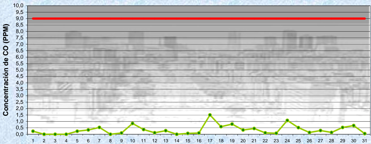
JULIO 2012 Concentración de CO- promedios de 8 hs
