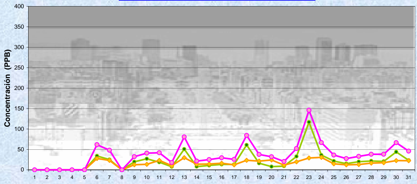
MARZO 2010 Concentración promedios de 8 hs De 0 a 8 Hs Estación La Boca ● NO ◆ NO2 ◆ NOx
