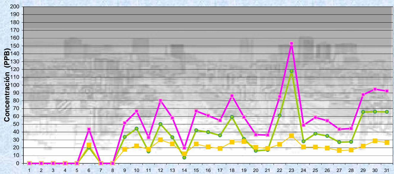
MARZO 2010 Concentración diaria Estación La Boca ● NO ■ NO2 ■ NOx
