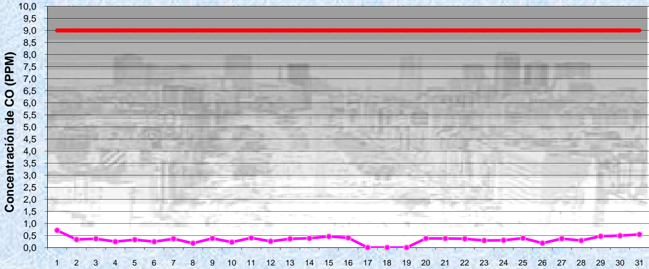
JULIO 2014 Concentración de CO- promedios de 8 hs
