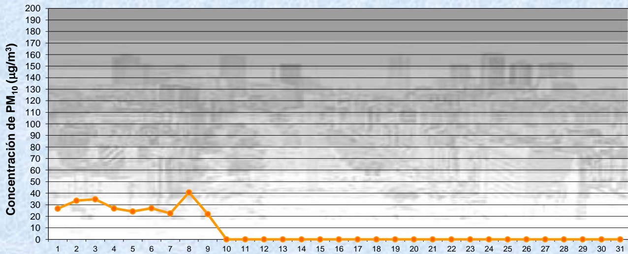
Estación Pque Centenario DICIEMBRE 2014 Concentración de PM 10 -Promedio de 8 Hs
