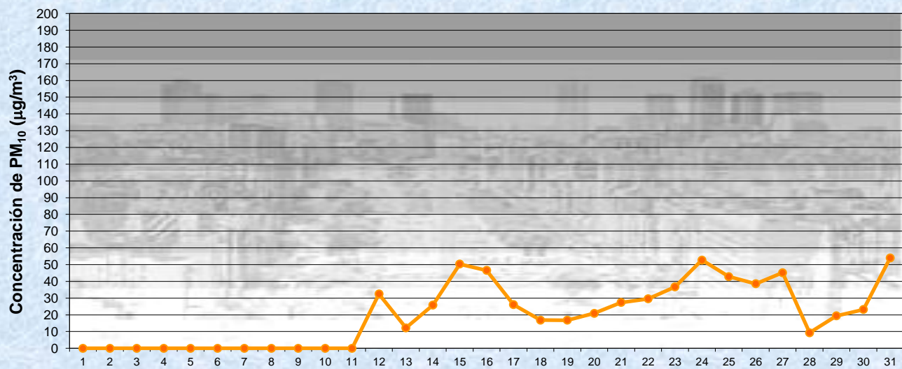
Estación La Boca ENERO 2015 Concentración de PM 10 -Promedio de 8 Hs PM10 de 16 a 24 hs
