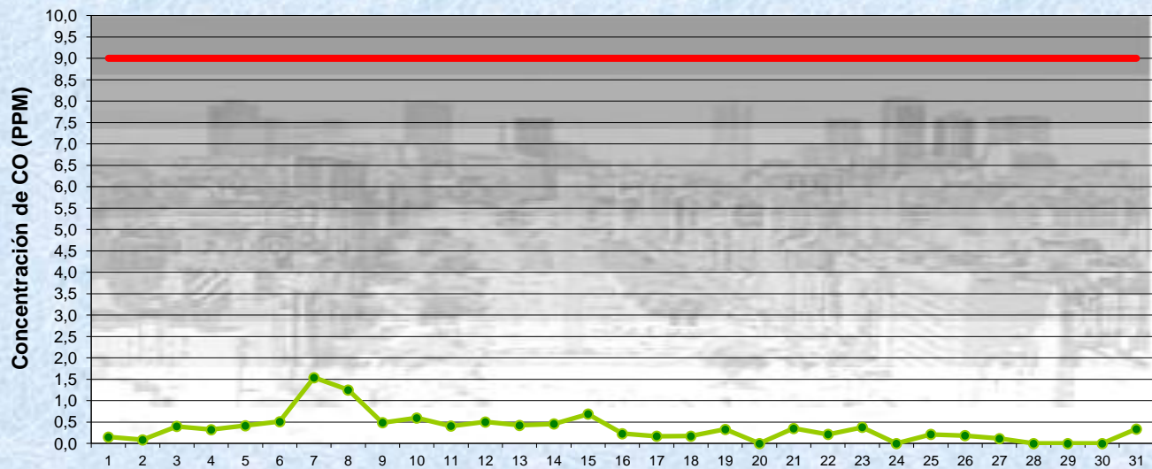
JULIO 2015 Concentración de CO- promedios de 8 hs
