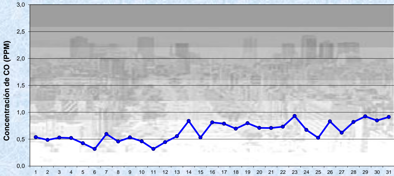
MARZO 2018 Concentración diaria de CO
