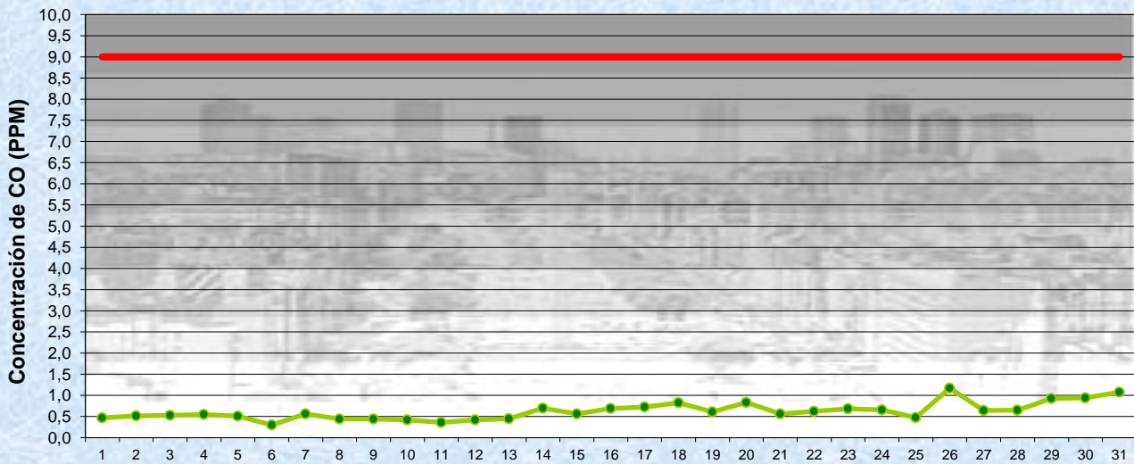
MARZO 2018 Concentración de CO- promedios de 8 hs
