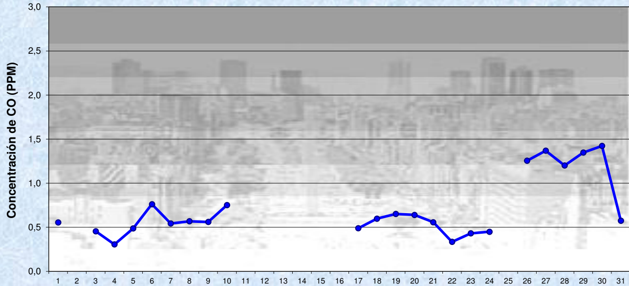
JULIO 2019 Concentración diaria de CO
