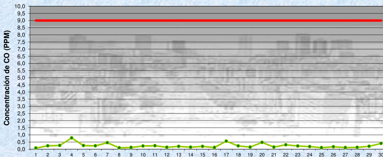
SEPTIEMBRE 2018 Concentración de CO- promedios de 8 hs
