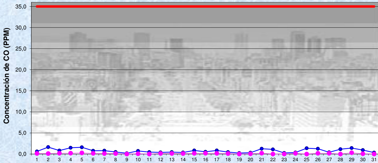
AGOSTO 2018 Concentración de CO- Máximos y mínimos en intervalos de 1 hora
